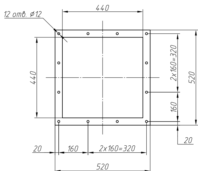
Фланец входа/выхода газа
