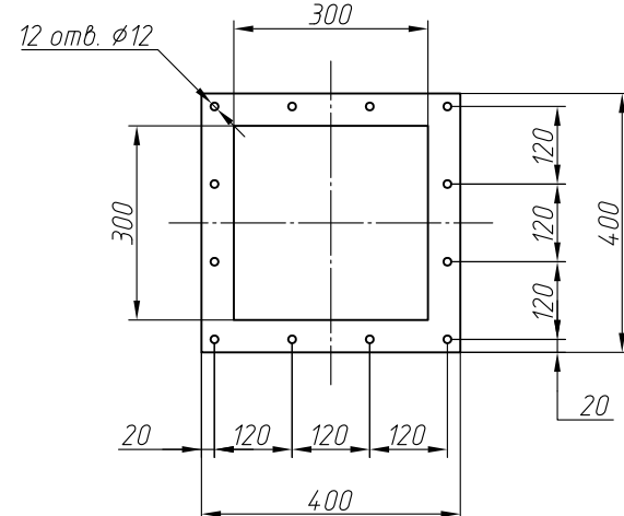
Фланец выгрузки пыли
